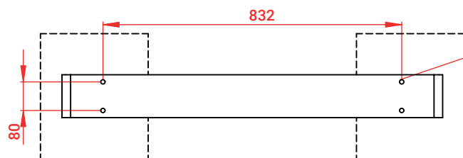
ROZSTAW OTWORÓW MONTAŻOWYCH (SKALA 1:15)
