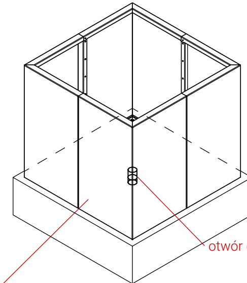
RZUT IZOMETRYCZNY
